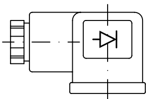
Connettori
