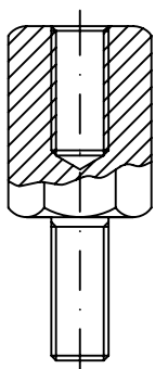
Raccordi M.F.
