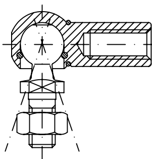
Snodi sferici 90°
