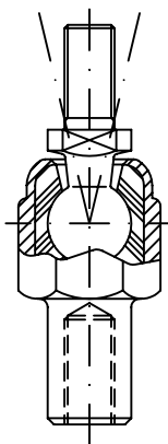
Snodi sferici assiali
